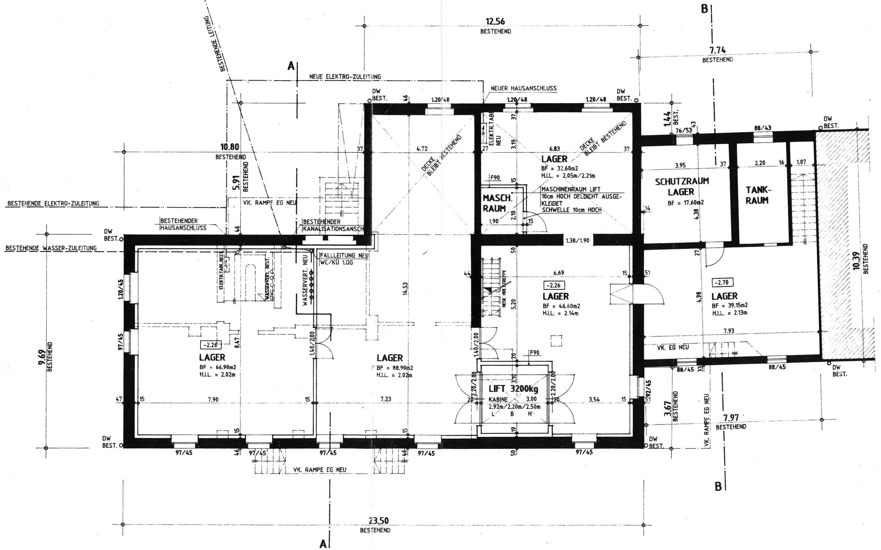
GRUNDRISS UNTERGESCHOSS
